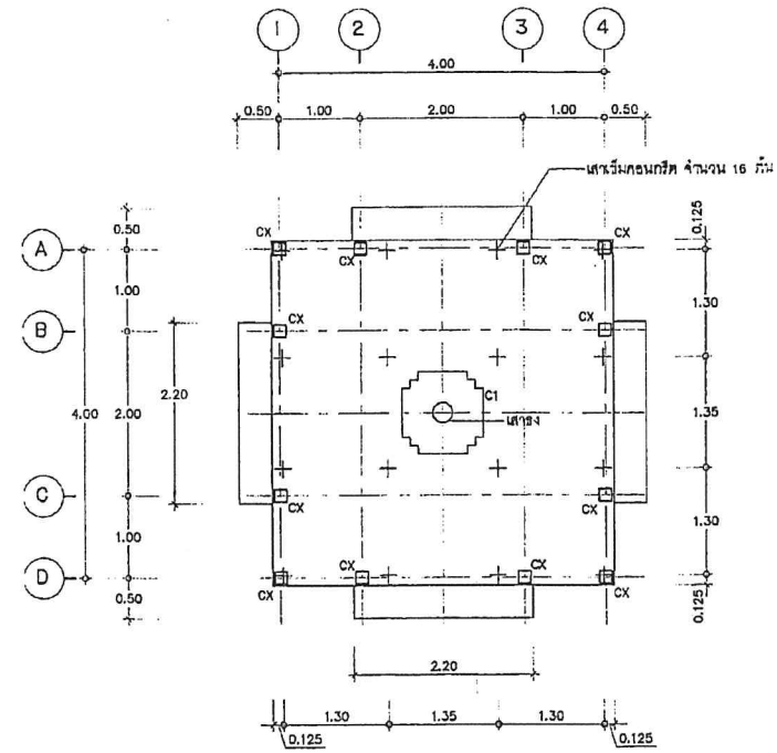
แปลนพื้น และฐานเสา
