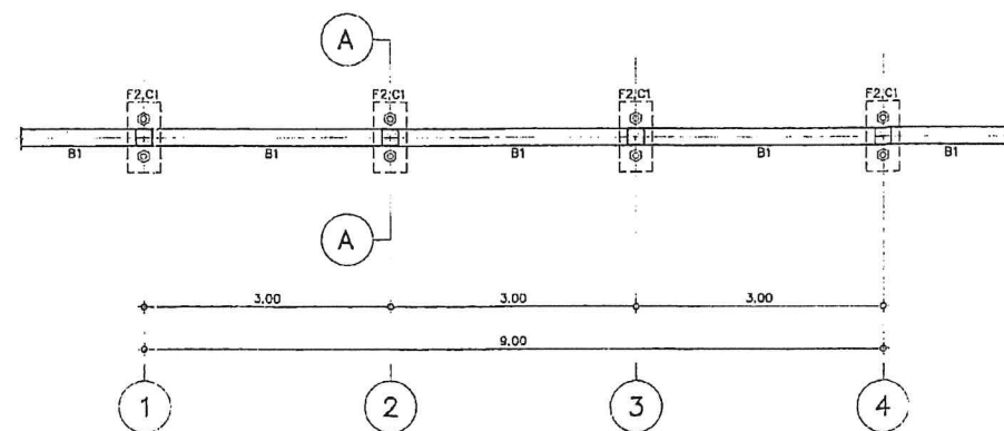
แบบแปลนขยายโครงสร้างรั้ว แบบ ก มาตราส่วน 1:50
