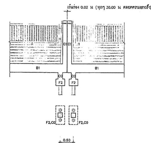
ขยายรอยต่อตัดขาดของรั้ว (ตัดขาดทุกๆ 30.00 ม) มาตราส่วน 1:50
