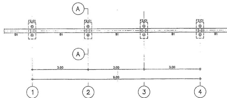
แบบแปลนขยายโครงสร้างรื้อ แบบ ข มาตราส่วน 1:50
