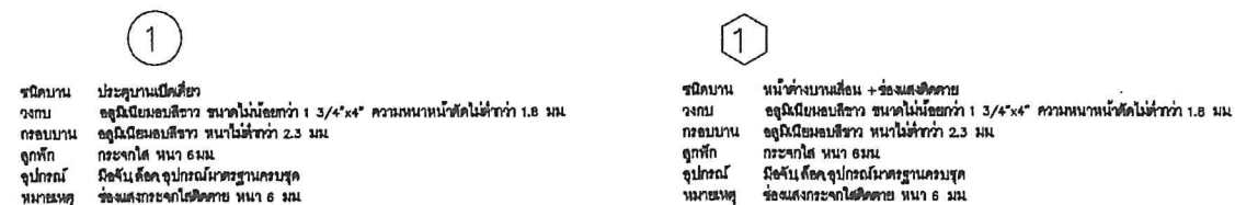
แบบขยายประตู - หน้าต่าง มาตรา ๑๑ 1 : 25
