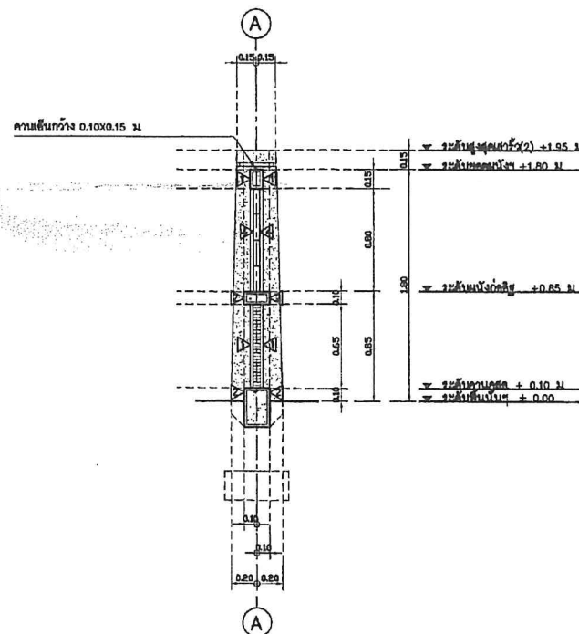
รูปตัดริ้วแบบ ข A
