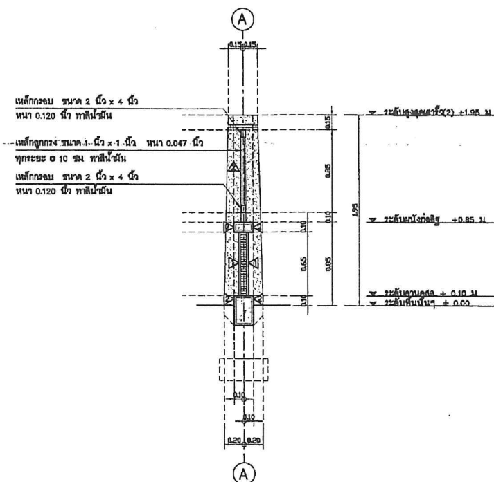
รูปตัดริ้วแบบ ก A มาตราส่วน 1 : 25
