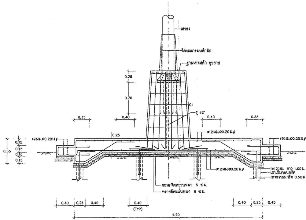
รูปตัดฐานเสา
