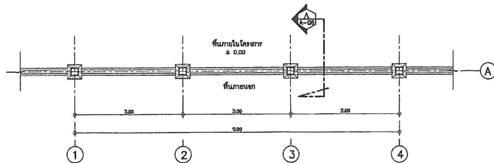
ผังพื้นริ้วแบบ ก มาตราส่วน 1 : 50
