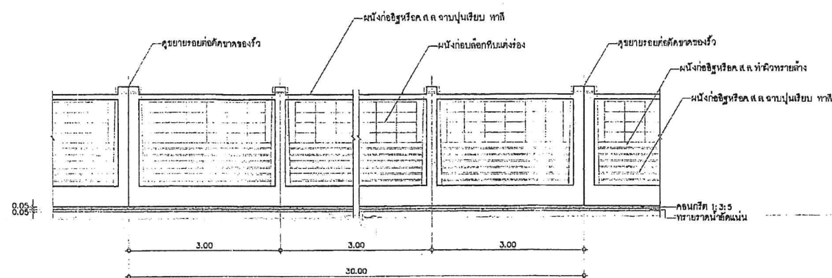
รูปด้านรื้อแบบ ข มาตราส่วน 1:50
