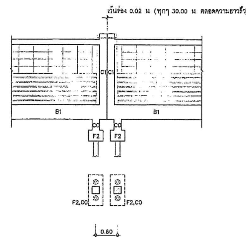
ขยายรอยต่อตัดขาดของรื้อ (ตัดขาดทุกๆ 30.00 ม) มาตราส่วน 1:50
