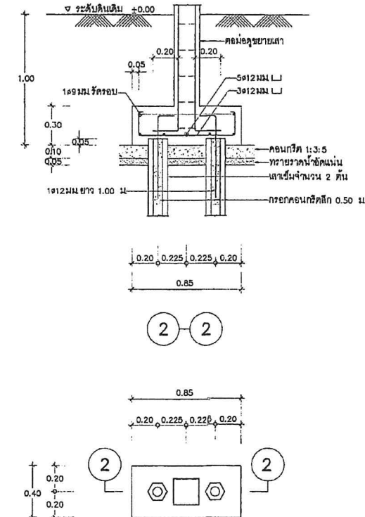
F2 มาตราส่วน 1:20
