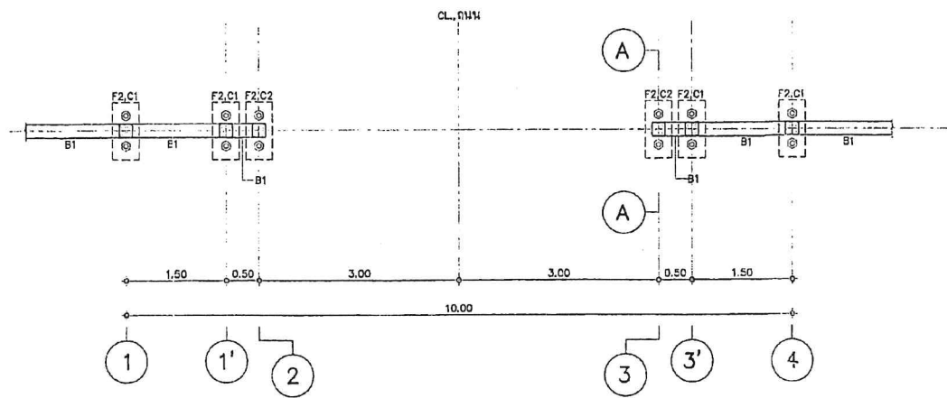
แบบแปลนขยายโครงสร้าง ประตูเข้า-ออก มาตราส่วน 1:50
