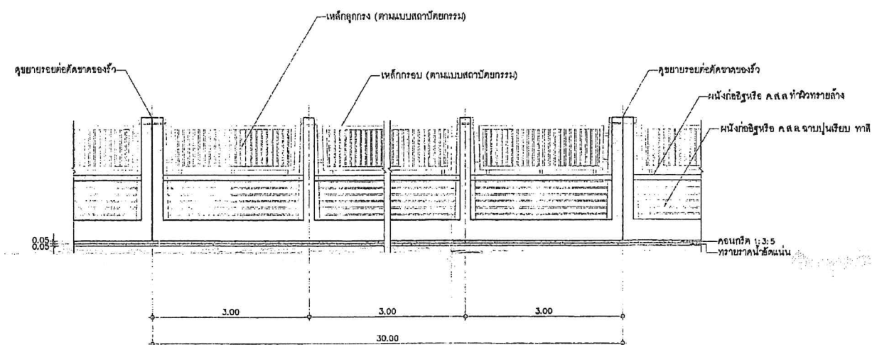
รูปด้านรั้วแบบ ก มาตราส่วน 1:50
