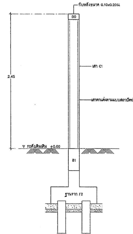
รูปตัด A มาตราส่วน 1:20
