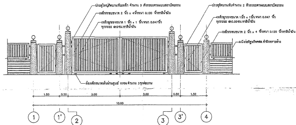
รูปด้าน ประตูเข้า-ออก มาตราส่วน 1:50
