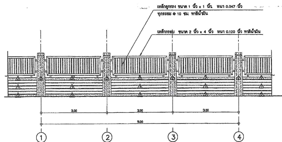
รูปด้านริ้วแบบ ก มาตราส่วน 1 : 50
