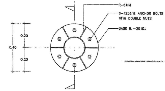
แบบขยายฐานเสาเหล็ก
