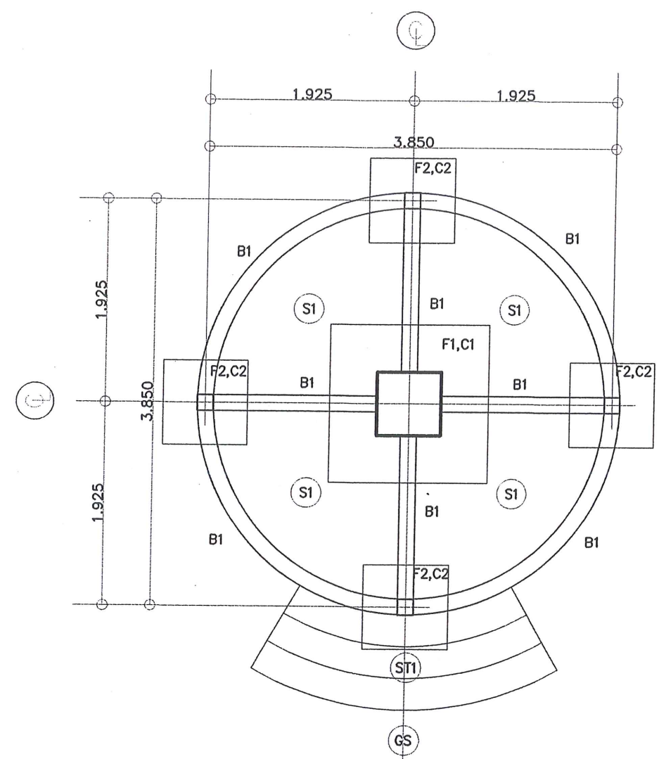
แปลนโครงสร้าง
