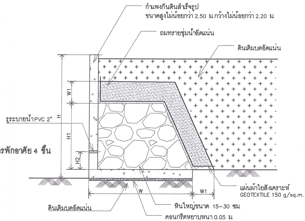
แบบขยายการติดตั้งกำแพงกันดิน TYPE 2 มาตราส่วน 1:50
