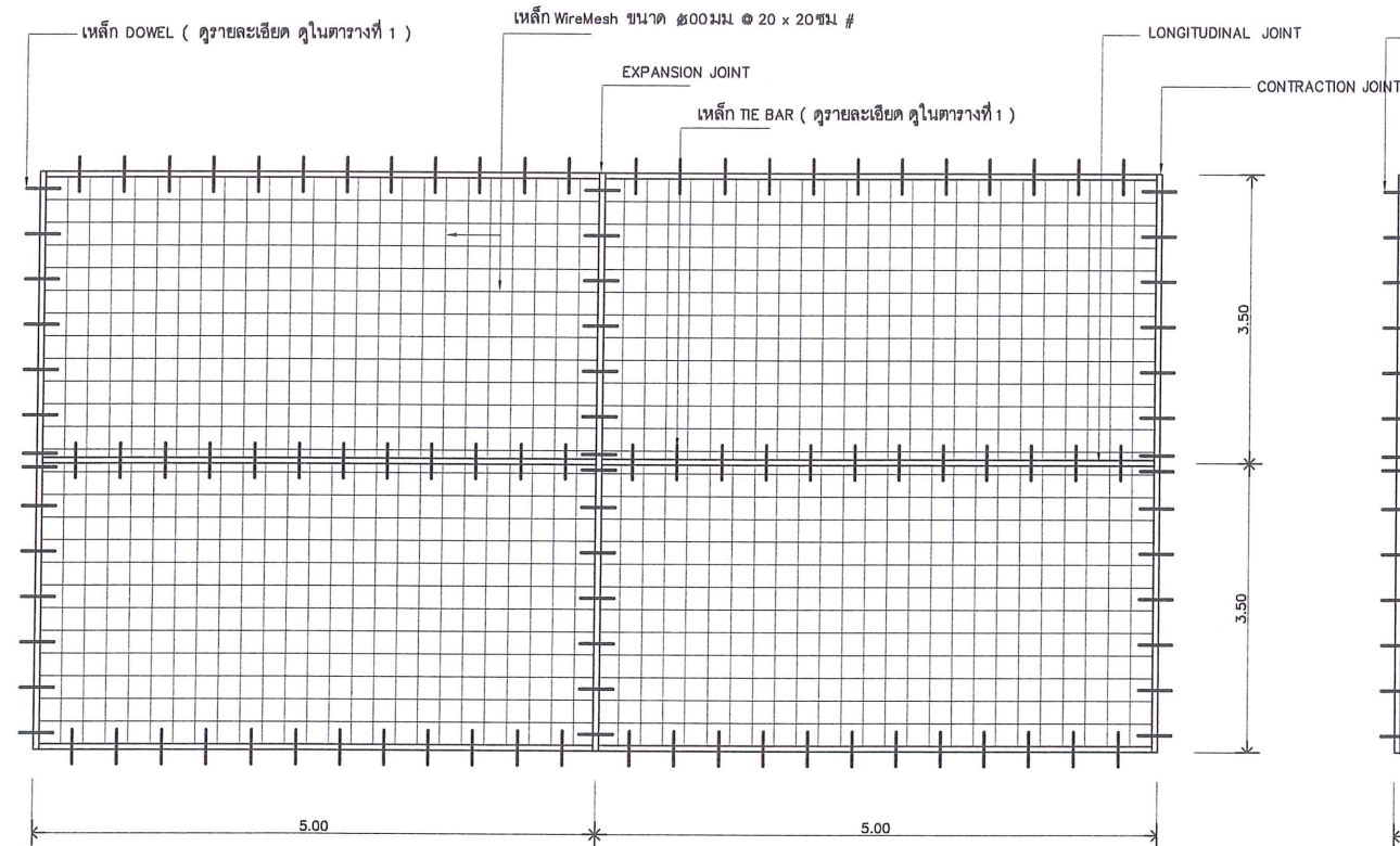
แปลนการวางตะแกรงเหล็ก ถนนกว้าง 7.00 ม. มาตราส่วน NTS.
