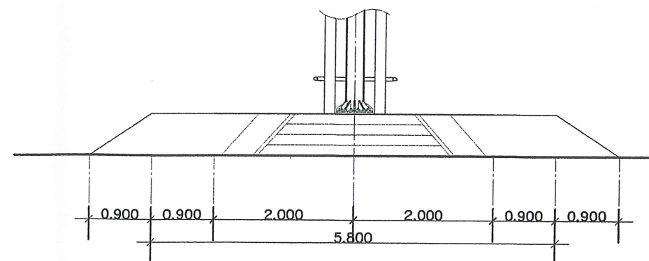
รูปด้านฐานเสาธง มาตราส่วน 1:50
