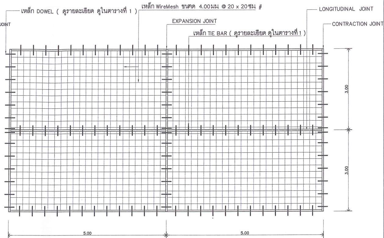
แปลนการวางตะแกรงเหล็ก ถนนกว้าง 6.00 ม. มาตราส่วน NTS.
