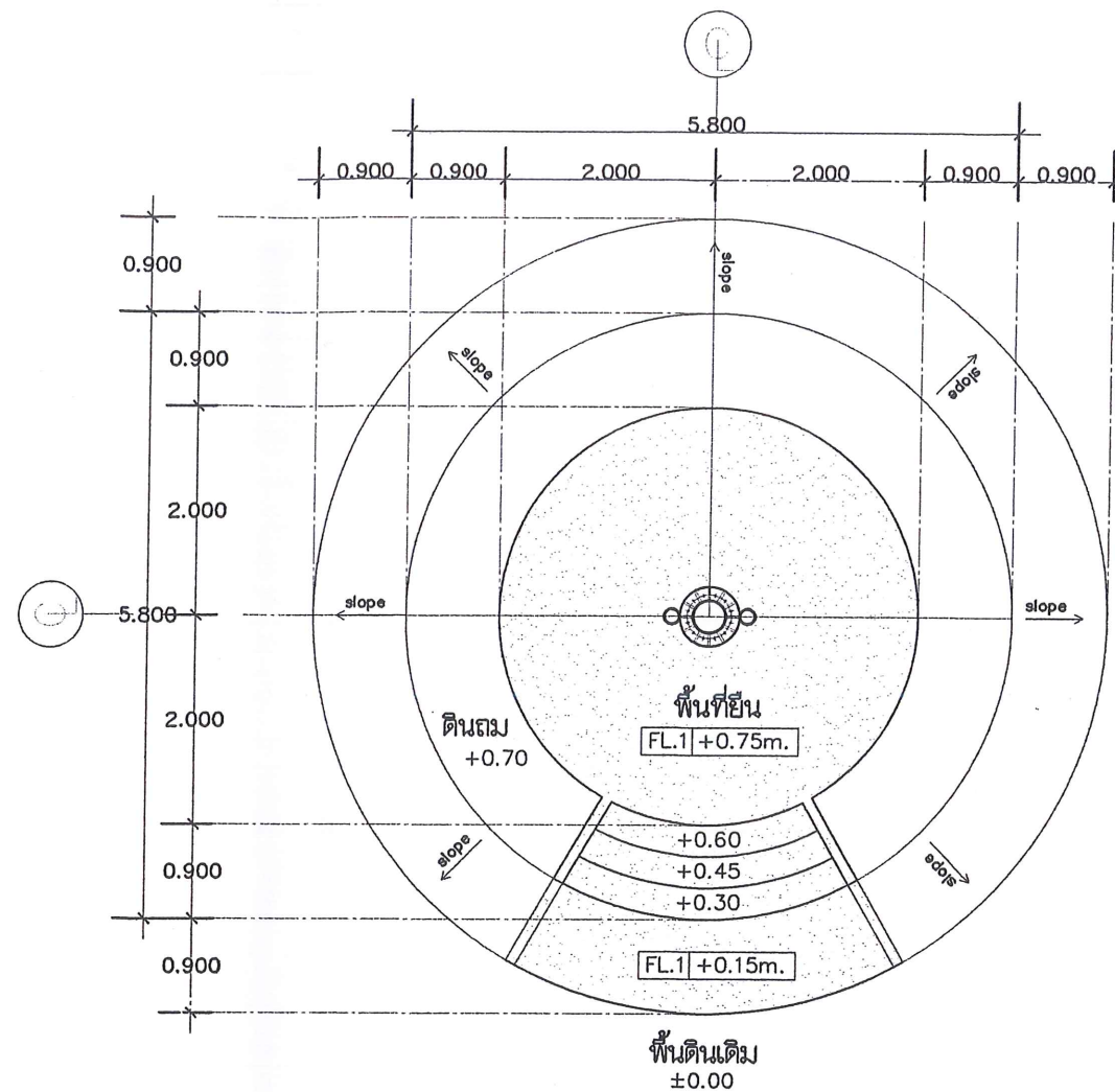
แปลนฐานเสาธง มาตราส่วน 1:50
