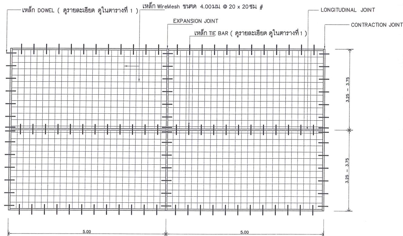
แปลนการวางตะแกรงเหล็ก ถนนกว้าง 7.50 - 6.50 ม. มาตราส่วน NTS.
