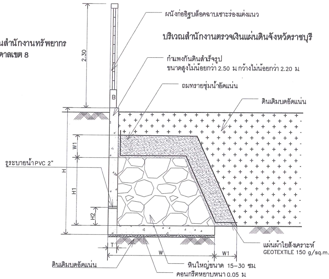
แบบขยายการติดตั้งกำแพงกันดิน TYPE 1 มาตราส่วน 1:50
