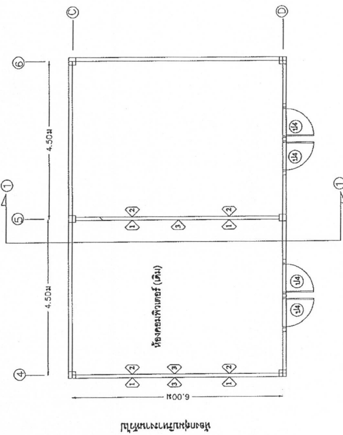
งานรีดคอนกรีตเสริมเหล็ก ชั้นที่ 2 GRID LINE 4 / C - D และบริเวณ GRID LINE 13 -14/ C - D (ห้องผู้ช่วยรายการกลุ่ม ตรวจสอบและทาสีผนังห้อง)
