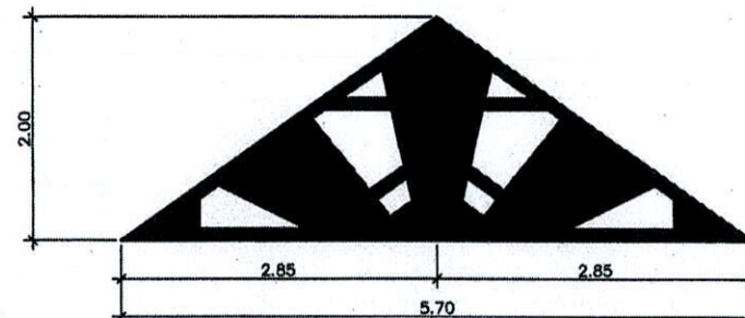
หน้าบัน แบบที่ 3
